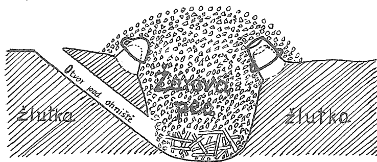
Čís. 5. Náčrtek pravděpodobného způsobu vypalování.
