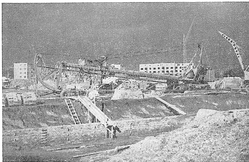
Staveniště sídliště na Struhlovsku — v popředí základy budovy jeslí pro 80 dětí, v pozadí obytné bloky.
