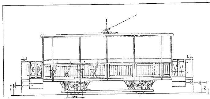
Schema pro nově budovaný salonní vyhlídkový vůz městských elektrických drah pro okružní jízdy Prahou.
