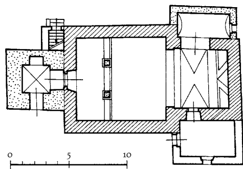
Plán kostela, převzato z knihy Bohumil Samek: Umělecké památky Moravy a Slezska, II. (1999)
